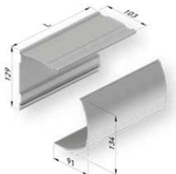
Set profile casetă ZIP 130
