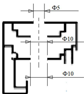
Găurire pentru montaj în cadru (în gol) Secțiune transversală profil
