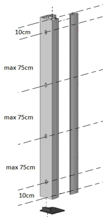
Distanța între găuri
