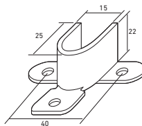
Soporte espiga 3 de orejas Number 3 support with flaps Support pivot 3 trous Supporto numero 3 con le orecchie
