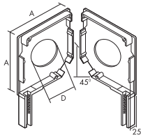
Testero con taladro central End cap with central hole Console avec trou central Fianco con foro centrale
