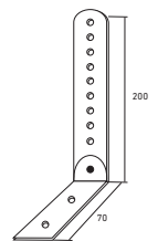
Escuadra Jabalcón Strut bracket Equerre jambe de force Staffa puntone
