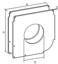
Placas contención 250/90 Safety plates 250/90 Plaques 250/90 Piastra di contenimento 250/90
