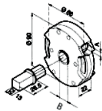
Cardán ACE 1:8 con final de carrera Gear ACE 1:8 with end of stroke Treuil ACE 1:8 avec fin de course Arganello ACE 1:8 con finecorsa
