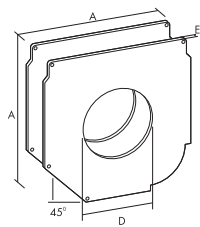
Placas contención 250/45 Safety plates 250/45 Plaques 250/45 Piastra di contenimento 250/45
