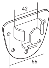
SopORTE de obra para rodamiento Support for traditional system & for ball bearing Support pour système traditionnel et pour roulement Supporto per sistema tradizionale per cuscinetto
