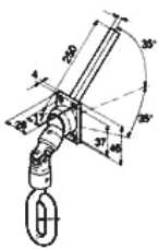
Snodo 45° con cáncamo zincado Joint 45° with zinc coated eye bolt Cardán 45° avec anneau zinc Snodo 45° con occhio zincato
