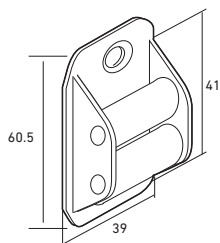
Pasacintas plástico modelo Norte rodillos plástico Plastic strap guide Norte type with plastic guide rollers Guide sangles plastique type Norte avec rouleaux plastiques Guidacinghia plastica tipo Norte con rulli in plastica
