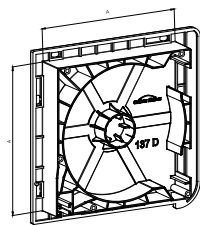
Juego de testeros ABS 137 curvo con rodamiento Set of ABS end caps 137 curved with ball bearing Jeu consoles ABS 137 courbe avec roulement Coppia fianchi ABS 137 curvo con cuscinetto
