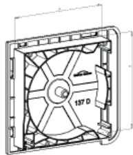
Juego de testeros ABS 137 curvo con espiga Set of ABS end caps 137 curved with pivot Jeu consoles ABS 137 courbe avec téton Coppia fianchi ABS 137 curvo con perno
