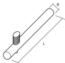
Cerrojillo de seguridad Small security lock Serrure de sécurité petite Serratura di sicurezza piccolo
