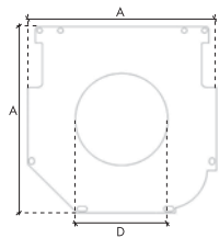
Placas contención 150/45 Safety plates 150/45 Plaques 150/45 Piastra di contenimento 150/45
