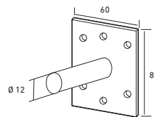
Placa con espiga para soporte L Square bracket with pivot for support L Plaque avec pivot pour support L Piastra con perno per supporto L
