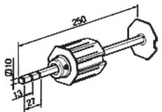
Cápsula regulable con perno 60 Ø10 Adjustable cap with pivot 60 Ø10 Embout réglable avec pivot 60 Ø10 Calotta regolabile con perno 60 Ø10
