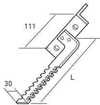
Lado corto soporte Cataluña F
