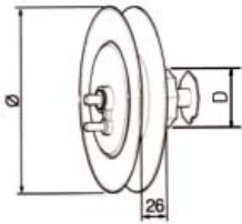
Disco reductor Reduction pulley Poulie démultiplicateur Puleggia riduttore
