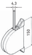
Recogedor Bandiera Mini Mini Bandiera coiler Enrouleur Bandiera Mini Avvolgitore Bandiera Mini
