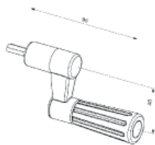
Manivela corta torno integral Short handle for integral rope winch Manivelle courte pour treuil à câble intégral Maniglia corta per arganello a fune integrale
