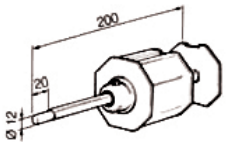
Cápsula regulable con perno 60 Ø13 - Ø12 Adjustable cap with pivot 60 Ø13 - Ø12 Embout réglable avec pivot 60 Ø13 - Ø12 Calotta regolabile con perno 60 Ø13 - Ø12
