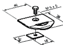
Muelle de bloqueo con tornillo y placa Stopper spring with screw and plate Ressort d'arret avec vis et plaquette Molla di arresto con vite e piastrina
